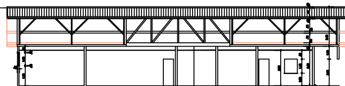
02 CORTE A-A Esc. 1:100
