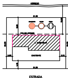
06 SITUACÃO Esc. 1:100
