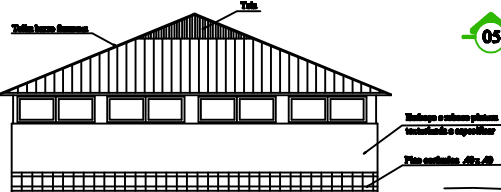
04 FACHADA LATERAL Esc. 1:100
