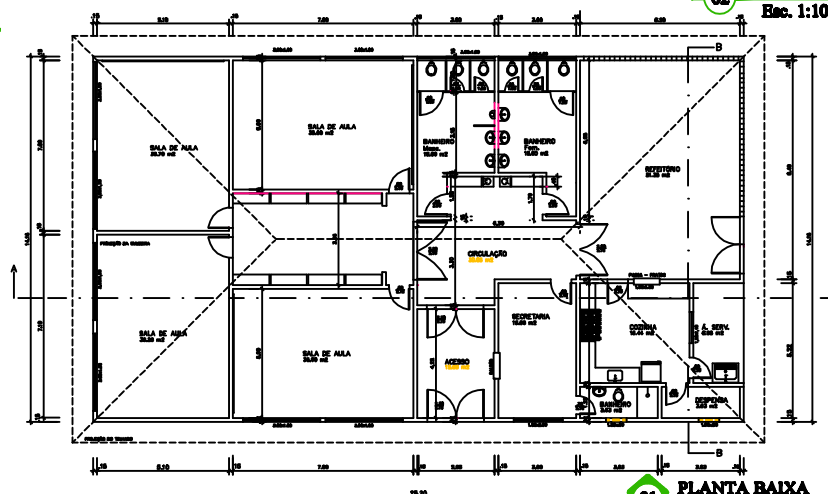
01 PLANTA BAIXA Esc. 1:100
