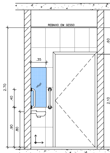
02 VISTA A - W.C. P.c.D. ESC. 1/25
