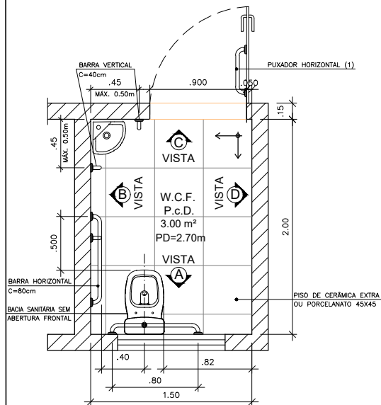
01 PLANTA BAIXA - W.C. P.c.D. ESC. 1/25
