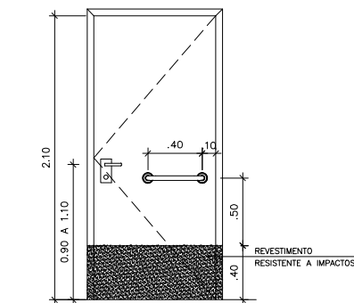
06 VISTA INTERNA PORTA - W.C. P.c.D. ESC. 1/25
