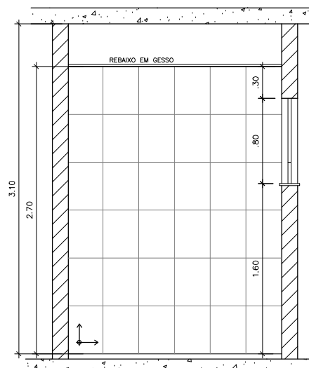
05 VISTA D - W.C. P.c.D. ESC. 1/25
